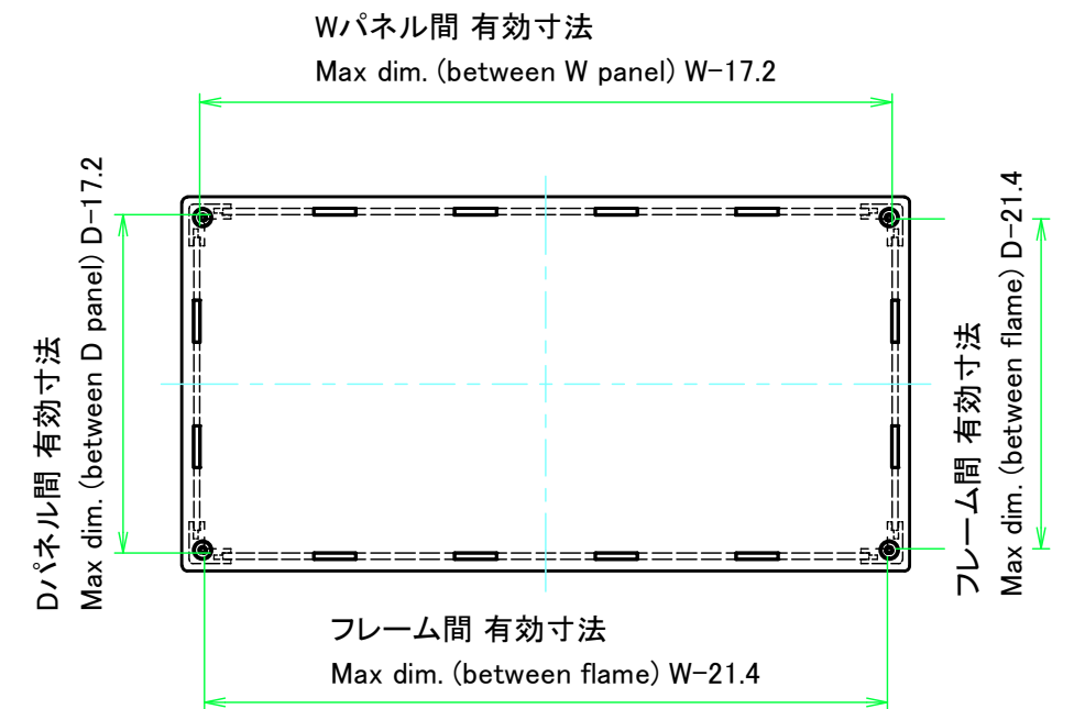
下カバー / Bottom cover
